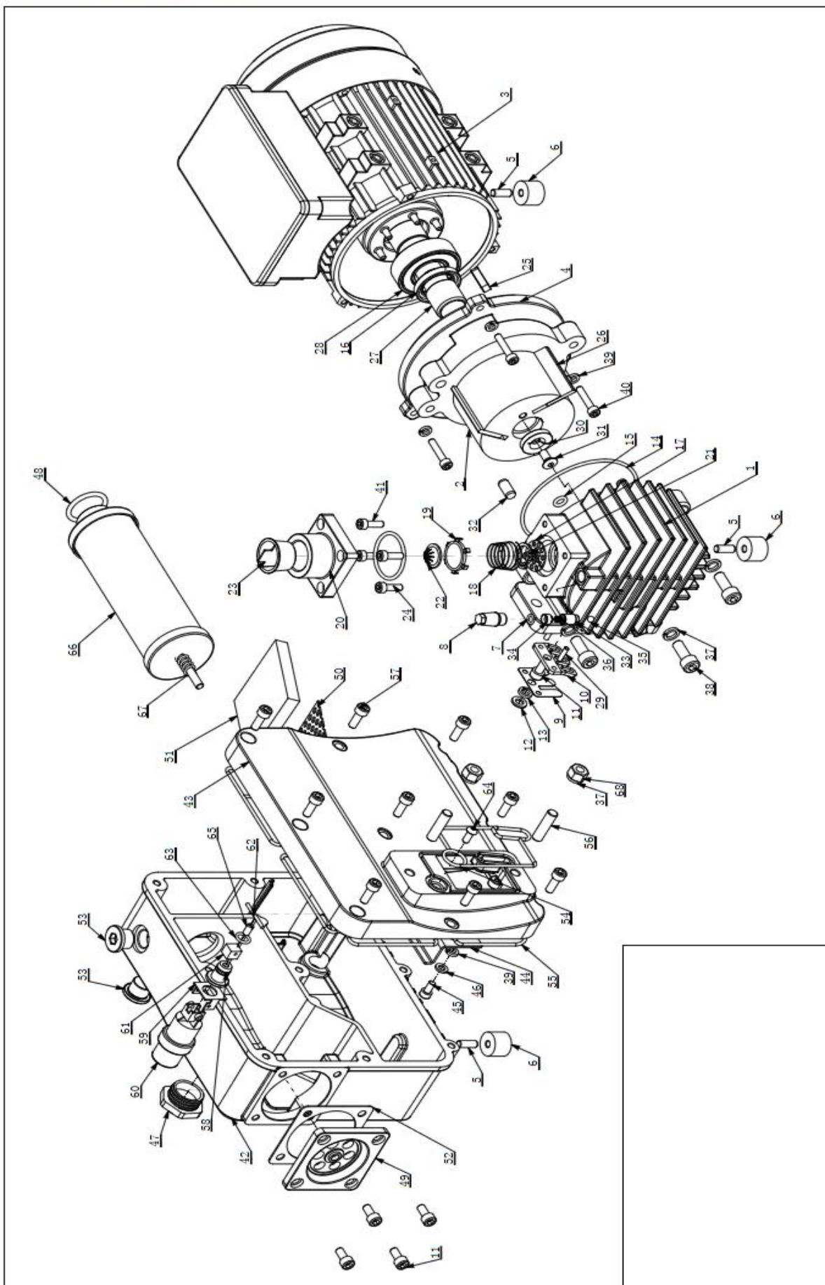
DLT.V0020真空泵分解图
